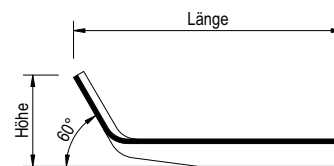
Maueranschlussstück WA Profil 8
