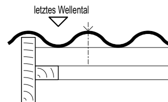
Ortgangausbildung mit freiem Überstand bei Wellplatten Profil 8
