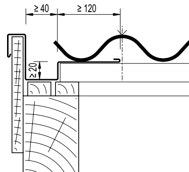
Ortgangausbildung mit untergedeckten Metallblechen
