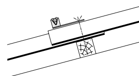
Dachleitungshalter für Blitzschutzleitung
