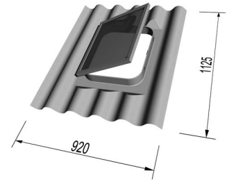
Wellfenster für Berliner Welle
