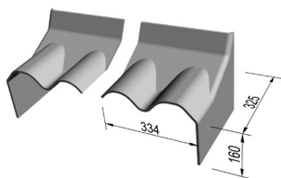
Wellgiebelwinkel Maueranschluss WGWK Typ links und rechts
