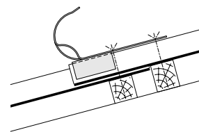
Dachhaken für Wellplatten
