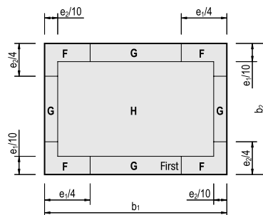
Überlagerte Dachbereiche bei freistehendem Gebäude
