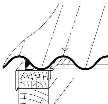
schräge Ortante Ausführung weglaufend
