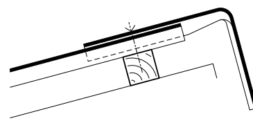
Pultfirst mit Wellpulthaube WP Profil 8
