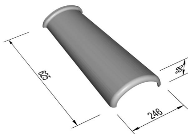
First-/Gratkappe GKK
