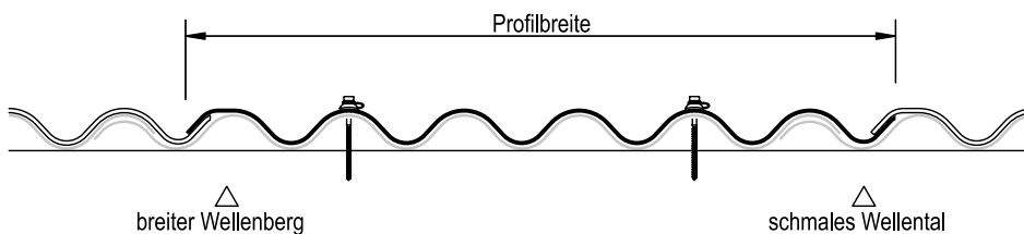
Profilform für Rechtsdeckendes (von links nach rechts) Formteil auf Wellplatte Profil 6¾
