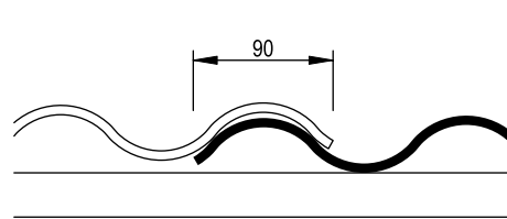
Seitenüberdeckung bei Eternit Wellplatten Profil 8
