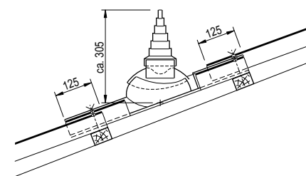
Kunststoff-Antennendurchgang
