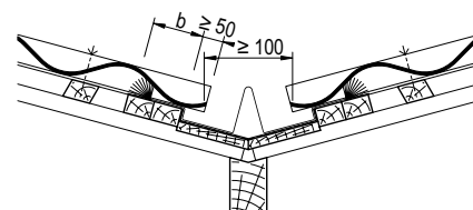
Kehlausbildung mit Steg im Kehlblech
