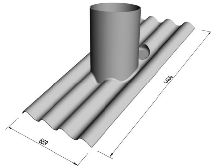
Rohrstutzen WS 5 – Ø 250 bis Ø 350
