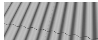
4. Nächste Reihe Wellplatten bis zum First mit Höhen- und Seitenüberdeckung verlegen
