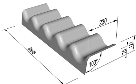
Traufenfußstück WE 230/70
