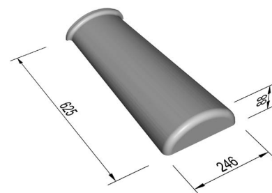
First-/Gratkappe GKK mit eingeformtem Schlussboden
