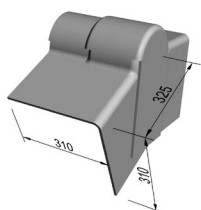
Einfacher Giebelwinkel Firstabschluss GWF für Wellfirsthauben WF 2-teilig, Ober- und Unterteil
