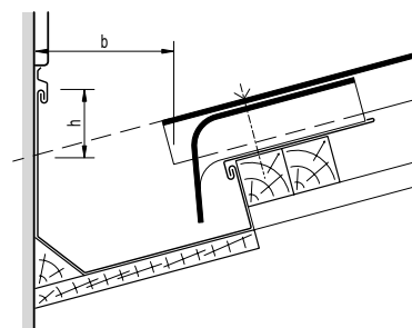
Wandanschluss firstseitig mit Rinne und Traufenfußstück WE
