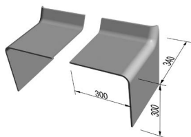
Einfacher Giebelwinkel Maueranschluss GWA Typ links und rechts
