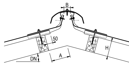
Firstausbildung als Kaltdachfirst WK bei Wellplatten Profil 8
