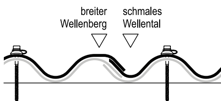
Seitenüberdeckung bei Linksdeckung der Wellplatten und Linksdeckenden Formteilen
