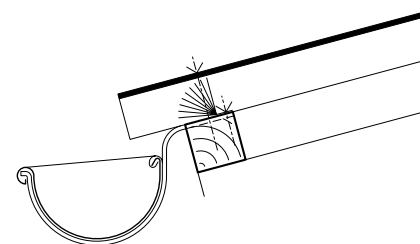
Traufenlüftungskamm TK
