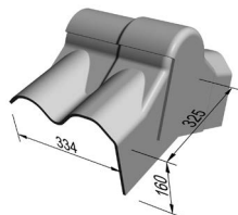
Wellgiebelwinkel Firstabschluss WGWFK für Wellfirstthauben WF 2-teilig, Ober- und Unterteil
