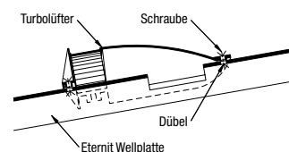
Einbauschema für Turbolüfter TL
