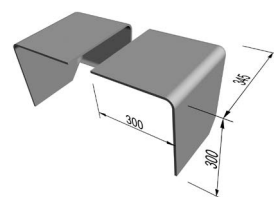
Einfacher Giebelwinkel Pultabschluss GWP Typ links und rechts
