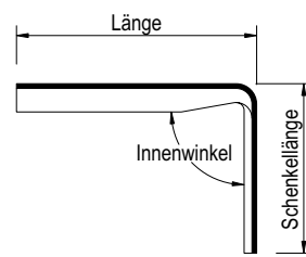
Wellpulthaube WP Profil 8
