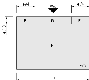
Windrichtung Traufseite
