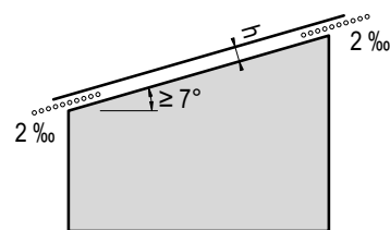
Lüftungsquerschnitte bei Pultdächern
