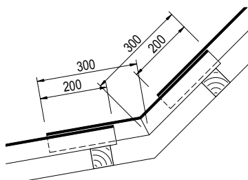
Wellübergangsstück WWS
