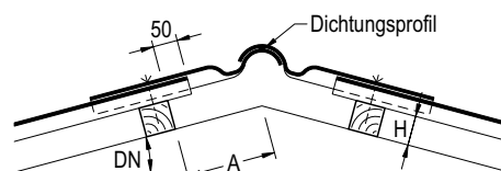
Firstausbildung mit Wellfirsthaube WF 2-teilig bei Wellplatten Profil 8
