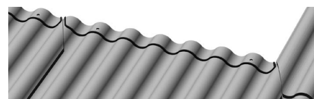
Lage der Dichtungsprofile im Bereich der Höhenüberdeckung bei Eternit Wellplatten Profil 6¾ und Profil 8
