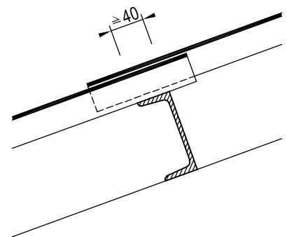
Mindestauflegerbreite bei Stahlträgern
