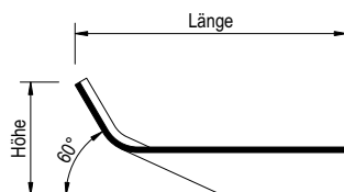
Maueranschlussstück WA Profil 5, Profil 6 und Berliner Welle
