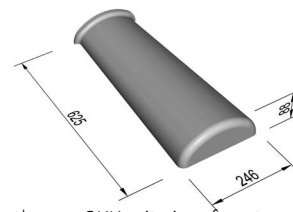
First-/Gratkappe GKK mit eingeformtem Schlussboden
