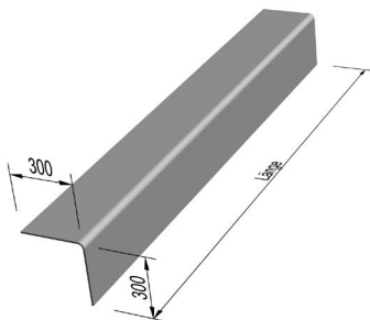
Einfacher Giebelwinkel GW 300/300
