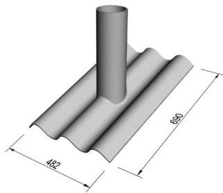
Rohrstutzen WS 5 – Ø 100 bis Ø 150
