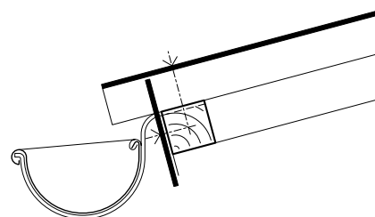
Traufenausbildung mit Traufenzahnleiste WST
