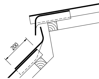
Ausführung mit Traufenfußstück WE und Maueranschlussstück WA
