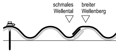
Seitenüberdeckung bei Rechtsdeckung der Wellplatten und Rechtsdeckenden Formteilen
