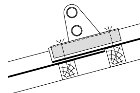
Schneefang mit 2-Rohr-System
