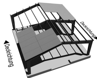
Die Abbildung zeigt ein Satteldach mit Linksdeckung der Wellplatten auf beiden Dachseiten
