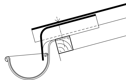
Traufenausbildung mit Traufenfußstück WE
