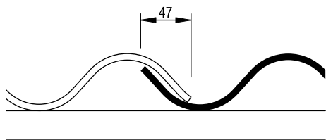
Seitenüberdeckung bei Eternit Wellplatten Profil 5, Profil 6 und Berliner Welle
