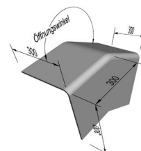
Einfacher Giebelwinkel Übergangshaube GWH Angabe des Öffnungswinkels > 180^\circ erforderlich
