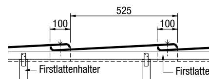
Verlege- und Befestigungsschema für First-/Gratkappe GKK
