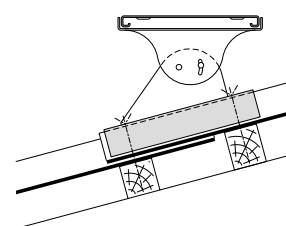
Laufroststütze für Wellplatten
