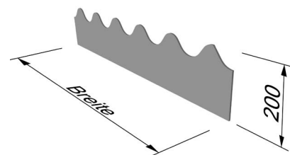
Traufenzahnleiste WST Profil 6
