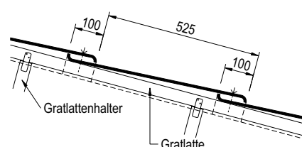
Verlege- und Befestigungsschema für First-/Gratkappe GKK
