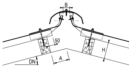
Firstausbildung als Kaltdachfirst WK bei Wellplatten Profil 5, Profil 6 und Profil 6 3/4
