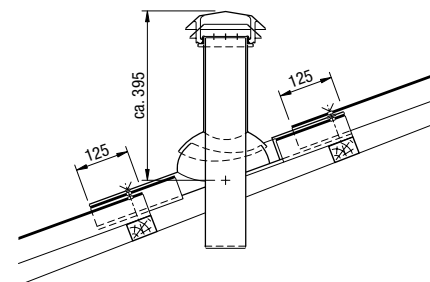
Kunststoff-Entlüfterstutzen
