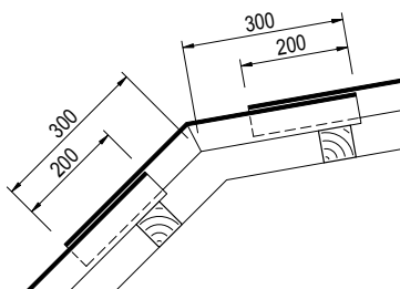
Wellübergangshaube WWH
