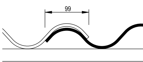
Seitenüberdeckung bei Eternit Wellplatten Profil 6¾ Kleiner Wellenberg muss überdeckt sein
